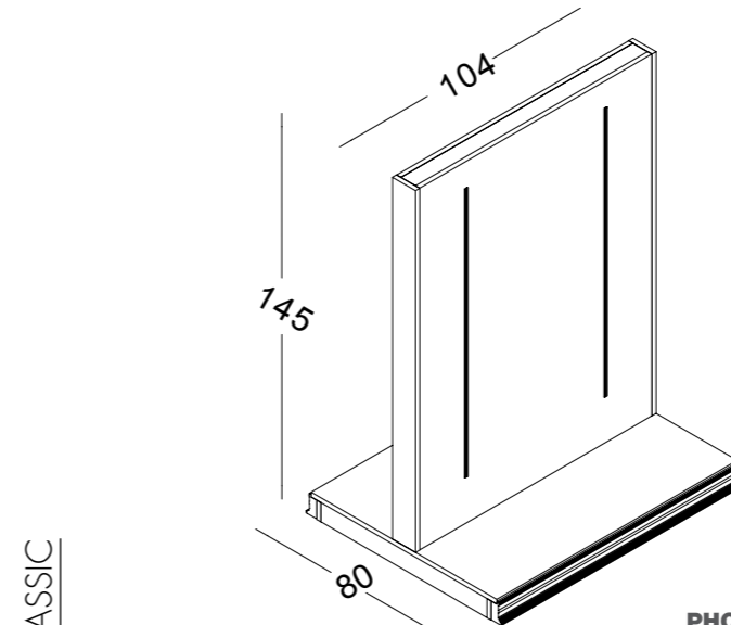
PHCLFV / L - N gondola bifacciale fondale vetrina+esposizione bifacial unit backdrop showcase+display in nobilitato in chipboard L104 x P80 x H145 cm
